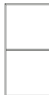
_art. 22/P _struttura pensile verticale 2 vani _cm L 59 - P 36 - H 118
