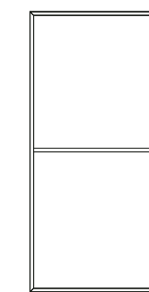
_art. 32/P _struttura colonna 2 vani _cm L 59 - P 36 - H 120,5
