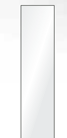
_art. 80/P _vetro trasparente per anta_art. 54/P _cm L 25,5 - SP 3 - H 106,5
