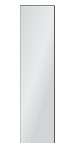
_art. 79/P _vetro satinato per anta_art. 54/P _cm L 25,5 - SP 3 - H 106,5
