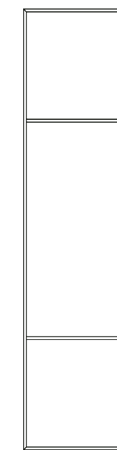
_art. 27/P _struttura colonna 3 vani _cm L 59 - P 36 - H 238,5
