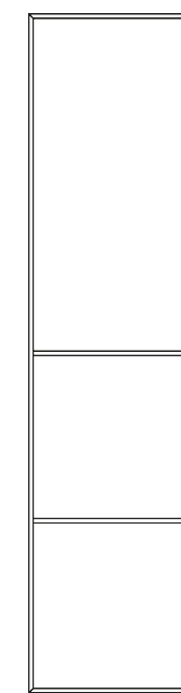
_art. 25/P _struttura colonna 3 vani _cm L 59 - P 36 - H 238,5
